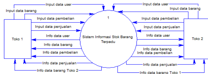
Gambar 1. Diagram Konteks
